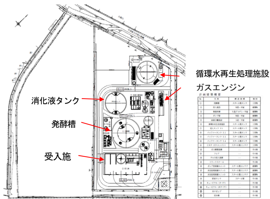
図 4-3 発電所図面
