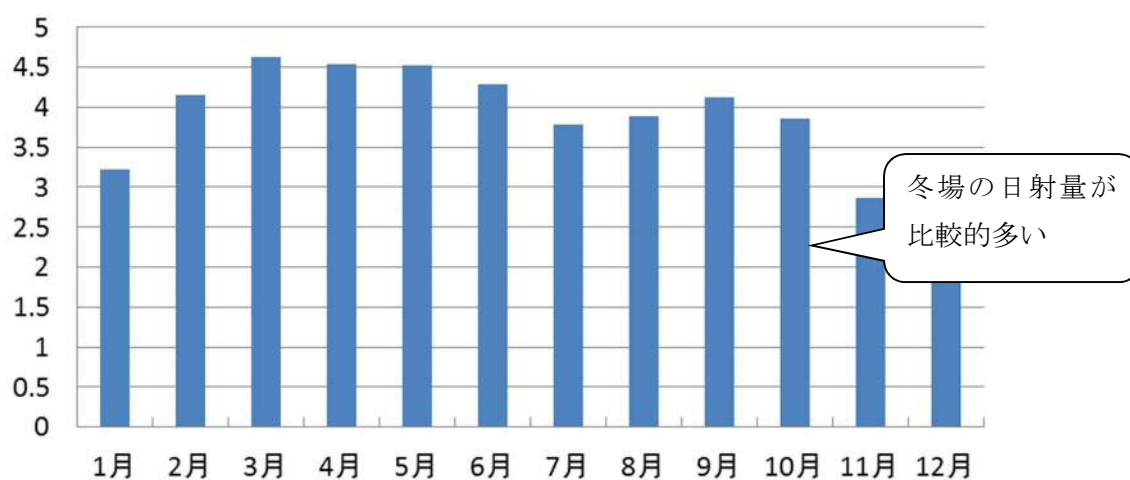
図 5.4-1 月平均斜面日射量[kWh/m2/day]
