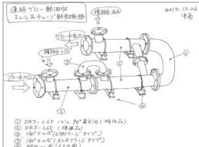
シェル&チューブ熱交製作ポンチ絵
